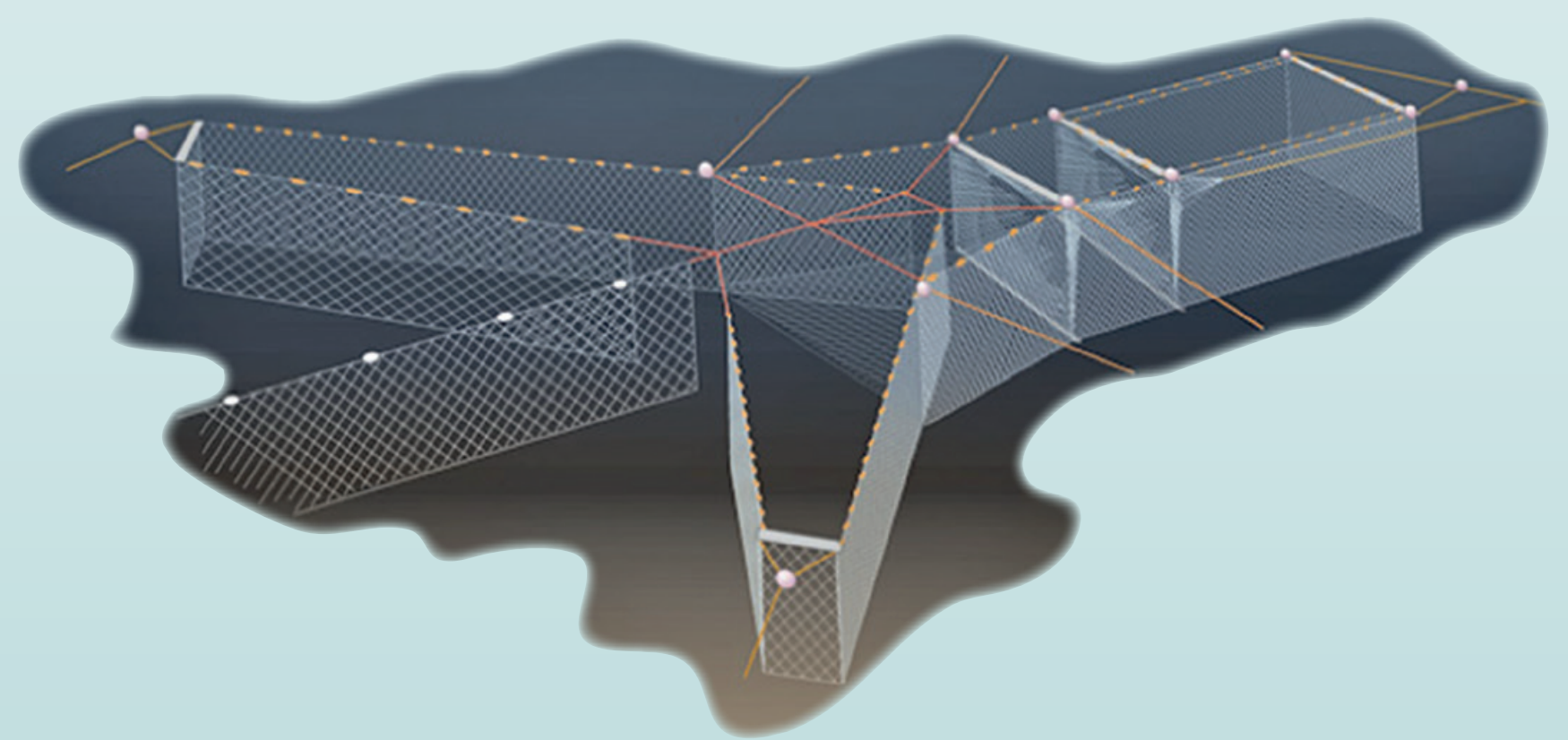
”Paunetti” eli päältä avoin rysä – pyyntikorkeus 2 m.
